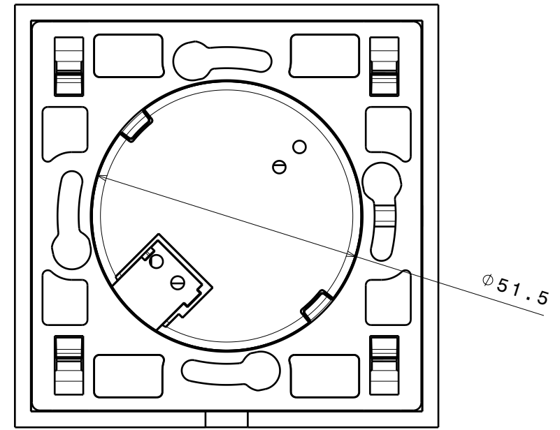
Vista dal basso Scala: 1:1
