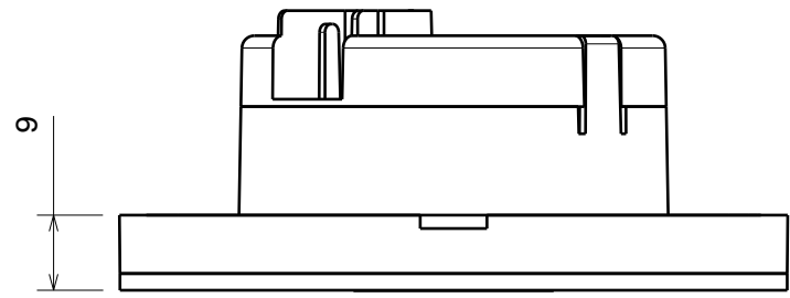
Vista da sinistra Scala: 1:1
